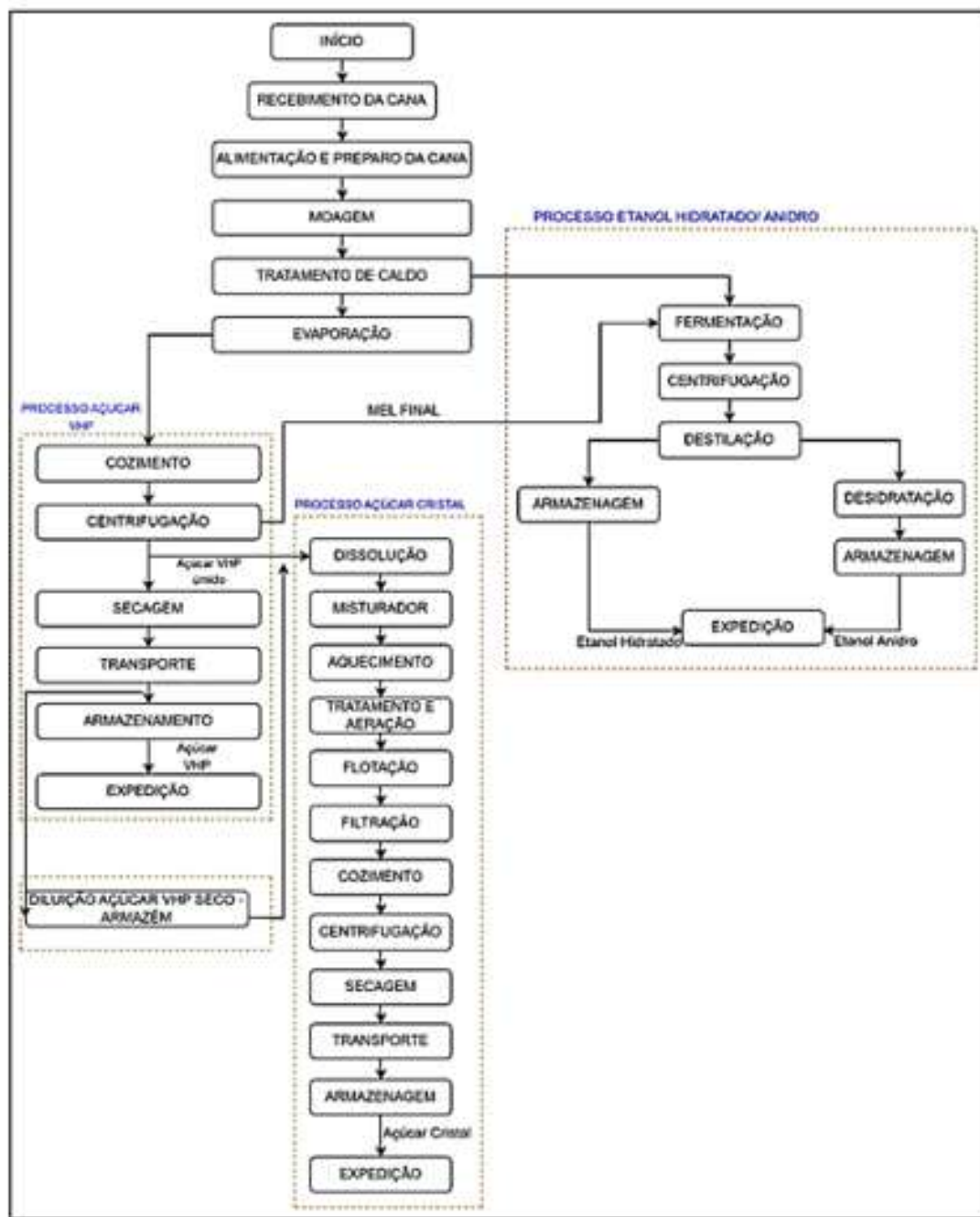
ANEXO 1 – FLUXOGRAMA DO PROCESSO INDUSTRIAL
